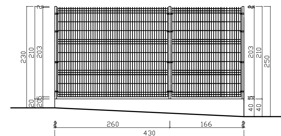
WIDOK ODCINKA A1-A2 (2x przęsło, 2x słupek) różnica wysokości ok. 20 cm
