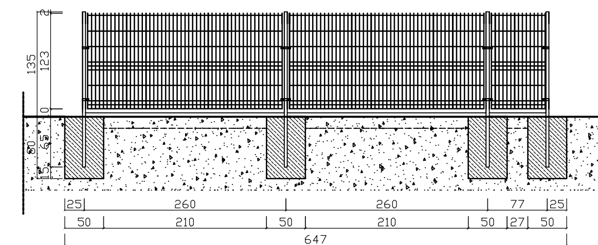
WIDOK ODCINKA B1-B2 (3x przęsło, 4x słupek)
