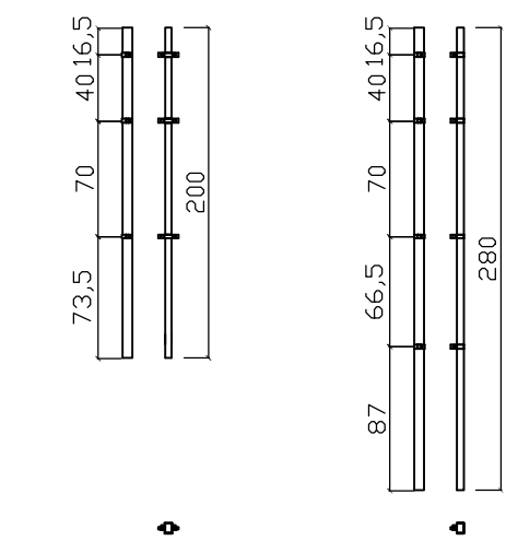
WIDOK BOCZNY SŁUPKÓW
