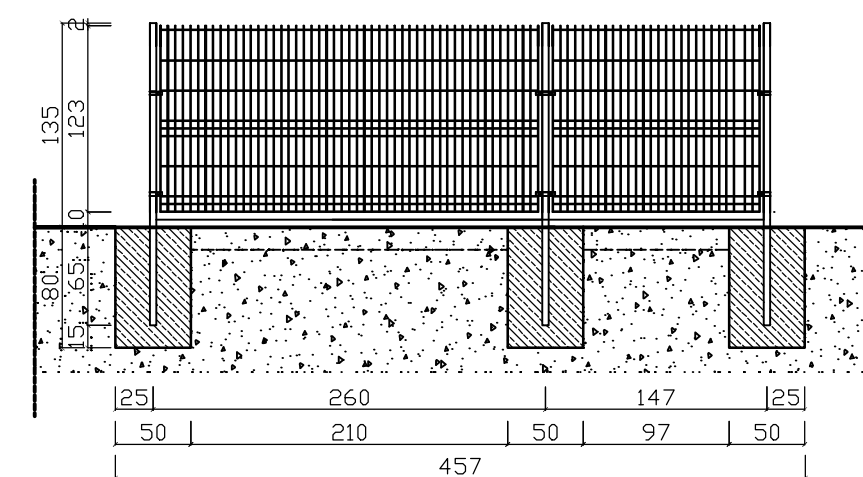
WIDOK ODCINKA B3-B4 (2x przęsło, 2x słupek)
