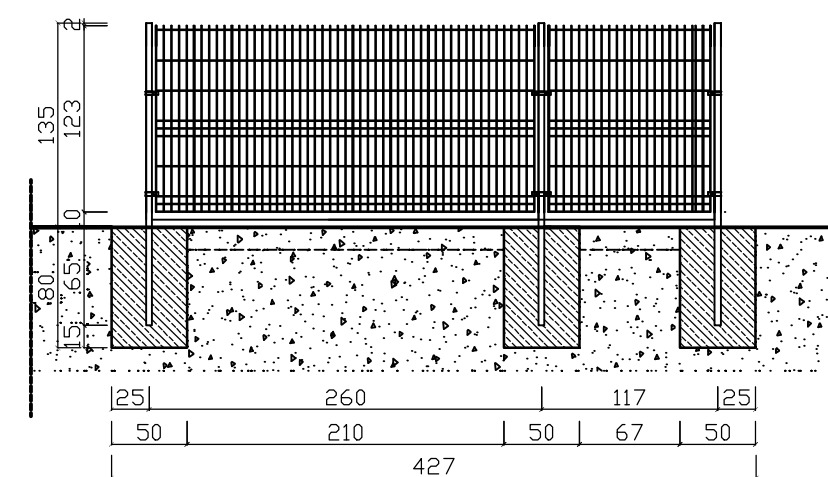
WIDOK ODCINKA B2-B3 (2x przęsło, 2x słupek)
